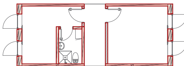
MODUL 6 MED BAD OG TOILET SAMT SKILLEVÆGGE I BEGGE SIDER
