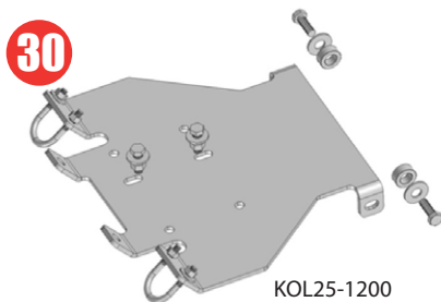
KOL25-1200
