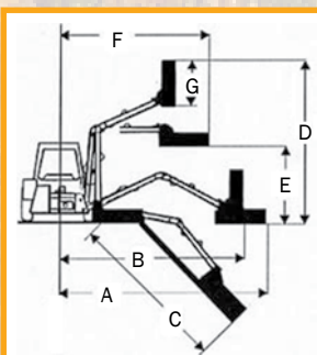
Snodo idraulico di sicurezza Hydraulic Safety brake away Articulation hydraulique de sécurité Hydraulisches Sicherheitsgelenk Articulación hidráulica de seguridad
