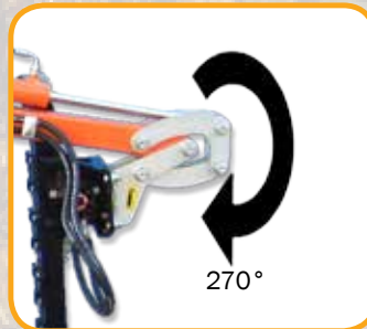
Snodo rotazione barra di taglio Tilting of the cutter bar Rotation de la barre de coupe Neigung des Scheidebalkens Articulación para rotación barra de corte
